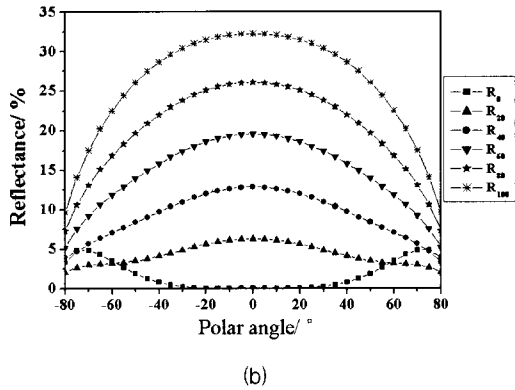
그림 6. (a) 수직과 (b) 수평 방향에서 6 계조별 시야각 의존성.
