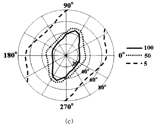
그림 7. 입사 파장별 등 명암대비비 곡선: (a) 480nm, (b) 550nm, (c) 630nm.
