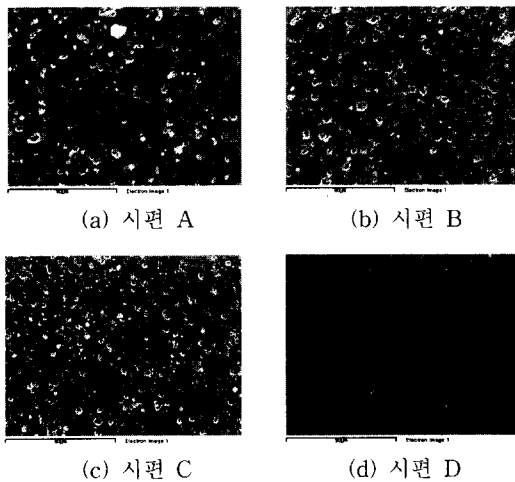
그림 4. 시편의 미세 조직 SEM 사진. Fig. 4. SEM photographs of samples.
