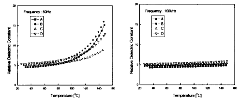
그림 5. 온도 변화에 따른 유전 상수 특성. Fig. 5. Relationship of relative dielectric constant and temperature.
