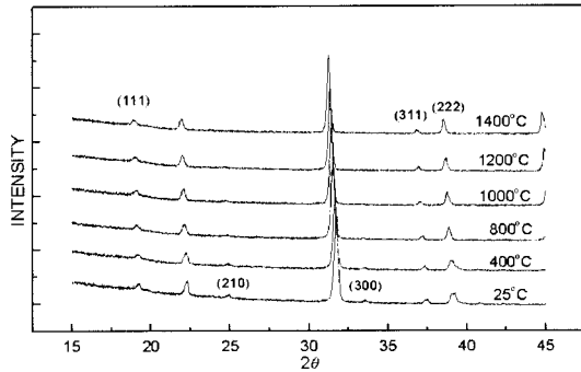
그림 5. 여러 온도에서 측정한 LMN의 X선 회절 패턴.
