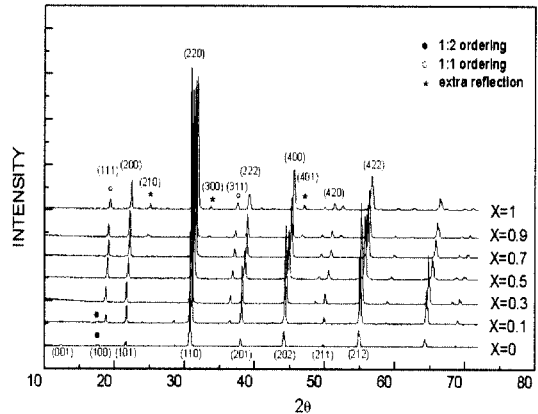
그림 1. 1450 °C에서 4시간 소결한 (1-x)Ba(Mg 1/3 Nb 2/3 )O 3 -xLa(Mg 2/3 Nb 1/3 )O 3 X선 회절패턴.
