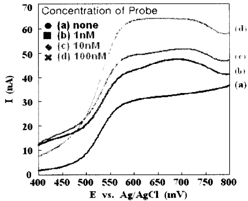
그림 9. Probe DNA의 고정화후 Hoechst 33258의 LSV. Fig. 9. Linear sweep voltammogram of Hoechst 33258 after immobilization of probe DNA.
