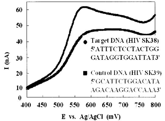
그림 10. Target DNA와 mismatched DNA의 hybridization후 Hoechst 33258의 LSV. Fig. 10. Linear sweep voltammogram of Hoechst 33258 after hybridization with target DNA and mismatched DNA.
