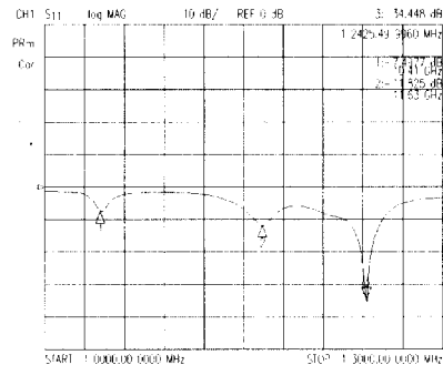
그림 10. 상온에서 비교용 금안테나의 반사손실. Fig. 10. Return loss for gold counterpart array at room temperature.
