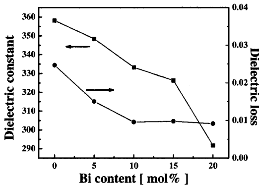
그림 6. 100 kHz에서 측정한 Bi 첨가량에 따른 유전상수 및 유전손실.
