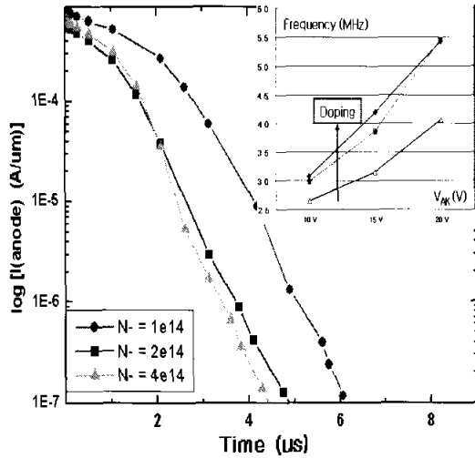
그림 8. N 영역에서 도핑농도 변화에 따른 anode 전류의 감쇄특성.
