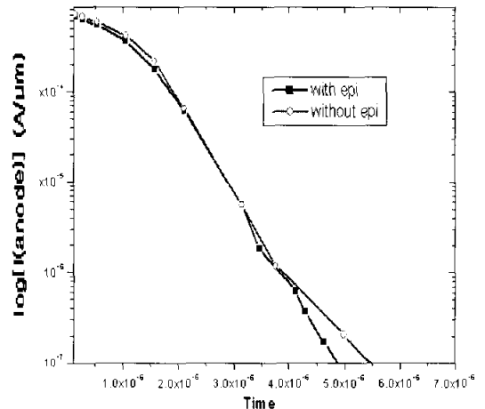
그림 4. EPI층의 적용에 따른 anode 전류의 turn off 특성. Fig. 4. Comparison of turn-off characteristics of anode current with application of EPI layer.
