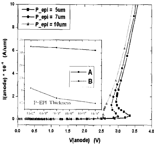
그림 5. P-EPI층의 두께에 따른 I-V 특성. Fig. 5. The I-V characteristics with variation of the thickness of P-EPI layer. (A; forward voltage drop (V) and B; latching current(amps/um))
