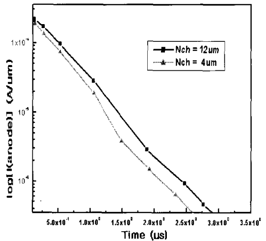
그림 6. N-채널 길이 변화에 따른 turn-off 특성. Fig. 6. Turn-off characteristics with variation of the N-channel length.
