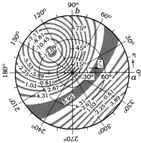
그림 4. [\bar{1}11] 방향으로 전기장을 가할 때 나타나는 단위길이당 단위전기장당 광행로길이 변화의 입체투영도( \times 10^{11} m/V).
