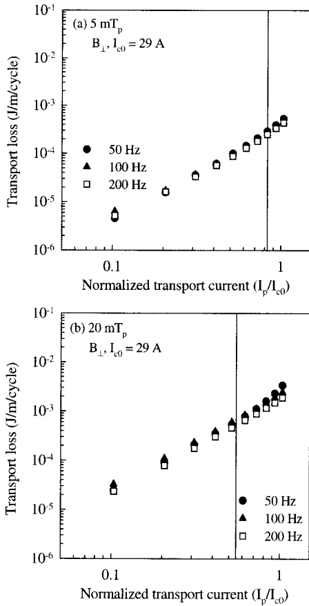
그림 6. Bi-2223테이프에 대한 통전손실의 주파수의 의존성.
