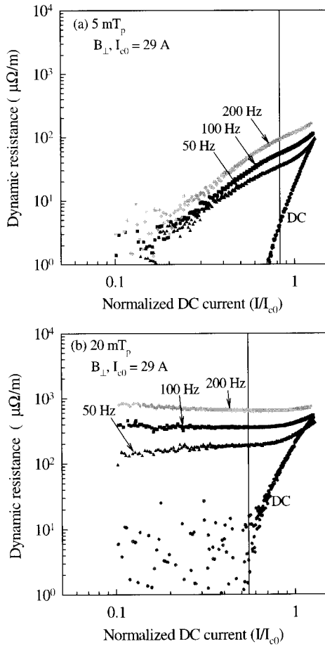
그림 4. Bi-2223테이프에 대한 동저항의 주파수의 의존성.
