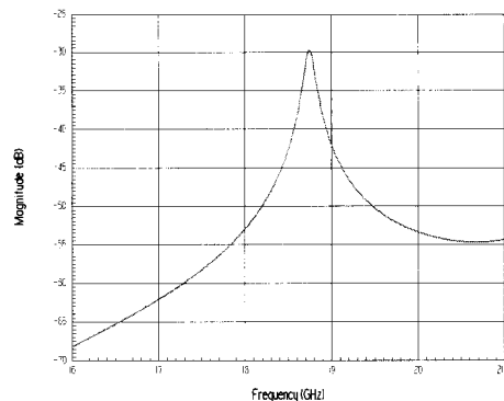
그림 3. HFSS를 해석한 coplanar stripline 공진기의 주파수 특성.
