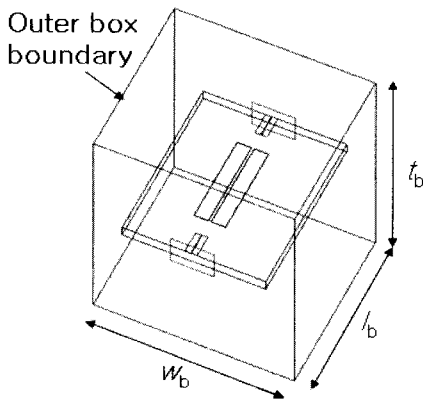
그림 4. Coplanar stripline 공진기 구조. Fig. 4. Structure of the coplanar stripline resonator.
