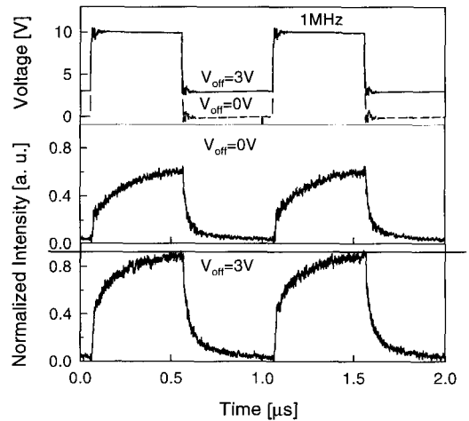
그림 3. 오프셋 전압 0 V 및 3 V에 대하여 피크 전압이 10 V인 펄스 전압을 인가하는 경우의 EL 신호 응답특성.
