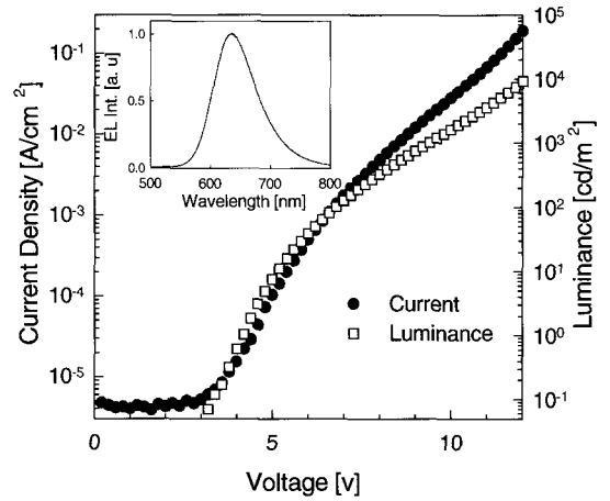
그림 2. 적색 유기 EL 소자의 전압-전류-휘도 특성 및 EL 스펙트럼.
