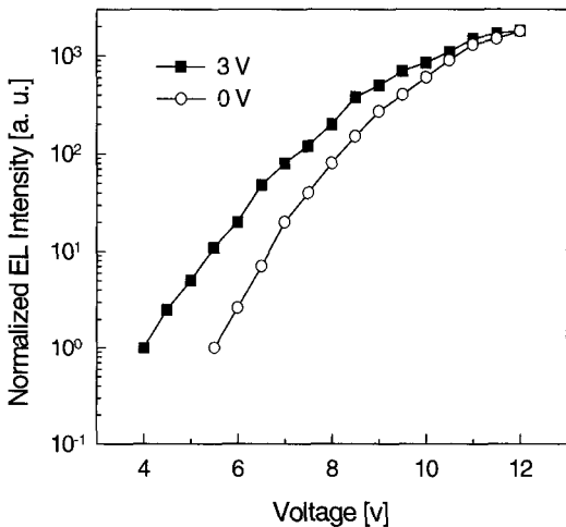
그림 5. 오프셋 전압 0 V 및 3 V에서의 인가전압에 대한 EL 신호 강도(주기 : 20 MHz).
