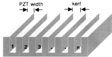
그림 1. 2-2형 압전복합재료의 구조.
