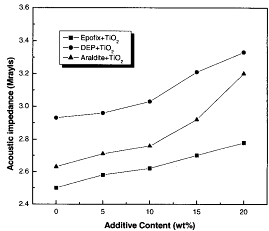
그림 4. 충전제의 첨가에 따른 음향임피던스 변화.
