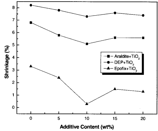
그림 3. 충전제의 첨가에 따른 수축률 변화.
