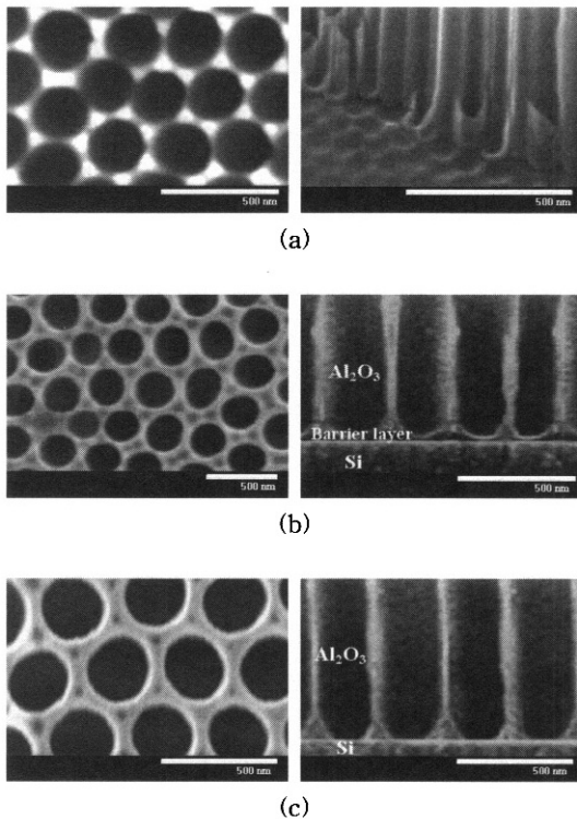
그림 5. 저농도 산(acid) 처리에 의한 베리어층의 제거. (a) 양극산화 후, (b) pore widening 후, (c) 저농도 산(acid)처리 후.
