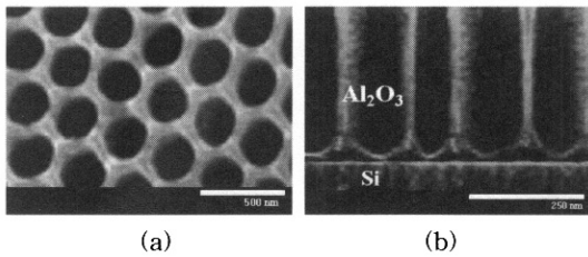
그림 4. Pore widening에 의한 미세기공의 변화. (a) pore widening 후 표면 (b) pore widening 후 단면
