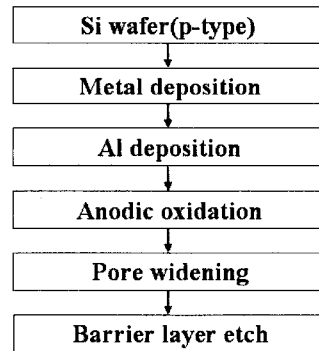
그림 1. 양극산화 공정도.
