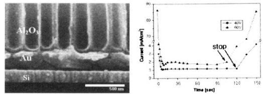
(b) 금속층이 있는 시편을 이용한 양극산화
