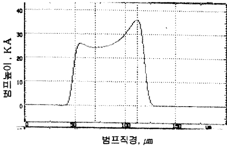
그림 5. 분수형 도금장비를 사용하여 형성된 솔더 박막의 두께. Fig. 5. Thickness of solder layer formed by fountain plating system.
