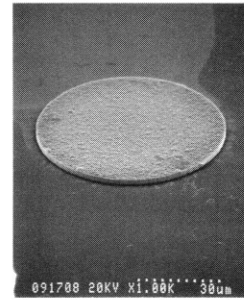
그림 6. 경사진 링구조의 도금장치에서 형성된 솔더 박막. Fig. 6. Solder layer formed by the tilted electrode ring plating system.
