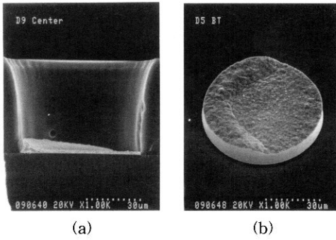
그림 4. 분수형 도금장비에 의해 형성된 솔더박막. (a) 단면도, (b) 평면도 Fig. 4. Solder layer formed by fountain plating system. (a) Cross section and (b) Plane surface
