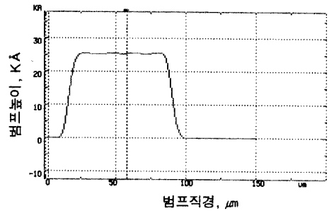
그림 7. 경사진 링구조의 도금장치에서 형성된 솔더 박막의 두께. Fig. 7. Thickness of solder layer formed by the tilted electrode ring plating system.
