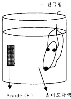
그림 3. 경사형 전극링 도금장치. Fig. 3. Tilted electrode ring plating system.
