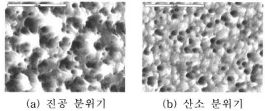
그림 3. 분위기 후열처리 공정에 따른 AZO 박막의 SEM 사진(60초 에칭).
