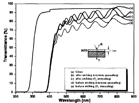
그림 6. 분위기 후열처리 공정에 따른 AZO 박막의 투과율.
