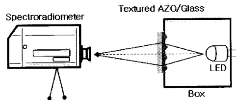
그림 1. 투과율 spectrum 측정을 위한 시스템 개략도.
