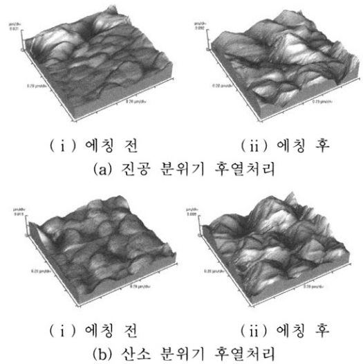
그림 4. 분위기 후열처리 공정에 따른 에칭 전 · 후 AZO 박막의 AFM 사진.
