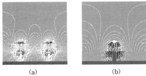
그림 8. HDE-IGBT에서 컬렉터 영역 부근의 전계 분포도. (a) HDE IGBT Type A (b) HDE IGBT Type B
