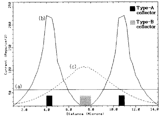
그림 7. 컬렉터 인근 영역에서 컬렉터 길이 방향에 따른 전자 전류 밀도 분포도. (a) 기존의 IGBT (b) HDE-IGBT Type A (c) HDE-IGBT Type B
