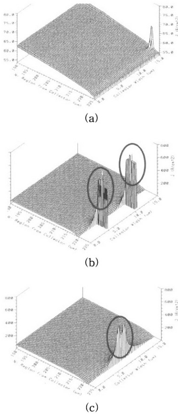
그림 6. 3차원 전자 전류 밀도 분포도. (a) 기존 IGBT (b) HDE-IGBT Type A (c) HDE-IGBT Type B
