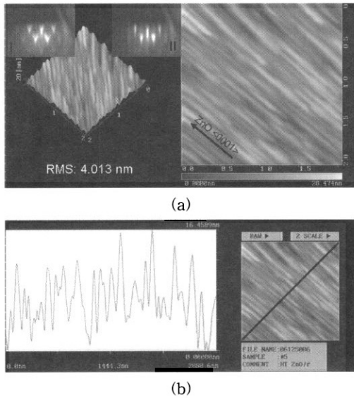
그림 6. (a) R-면 사파이어 기판 1시간 성장된 (11-20) ZnO 박막의 AFM 사진. 삽입된 RHEED 사진 I, II는 각각 10분 및 1시간 성장 시의 패턴을 보여준다. (b) <0001>에 수직인 방향의 대각선으로의 표면 라인 스캔 결과.
