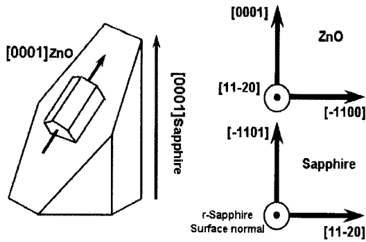
그림 4. ZnO 박막과 R-면 사파이어기판과의 에피택셜 방향관계를 보여주는 개략도.
