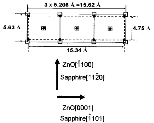
그림 5. 결정된 에피택셜 관계에 대한 R-면 사파이어와 a-면 ZnO의 양이온 위치를 보여주는 개략도. 채워진 원은 Al 원자 위치, 점선은 R-면 사파이어 단위격자를 나타내며, 빈 사각형은 Zn 원자 위치, 실선은 ZnO a-면 단위격자를 나타낸다.
