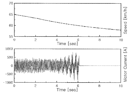
그림 4. 고장시의 전동기 출력 전류. Fig. 4. Motor output current in case of fault.
