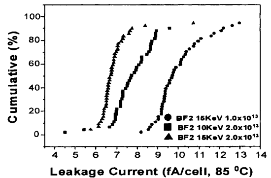
그림 5. 64 K 셀 어레이를 이용하여 85 °C에서 측정된 누설전류의 누적분포. Fig. 5. Cumulative distribution of leakage current in 64 K cell array, at 85 °C.
