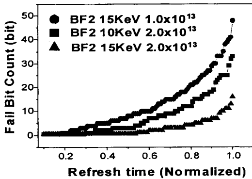
그림 2. 평면구조 P-MOS DRAM 셀에서 커패시터 V_T 이온주입 조건에 따른 refresh 시간 분포. Fig. 2. The measured refresh time distribution with different condition of capacitor V_T implant for planar P-MOS DRAM cell.
