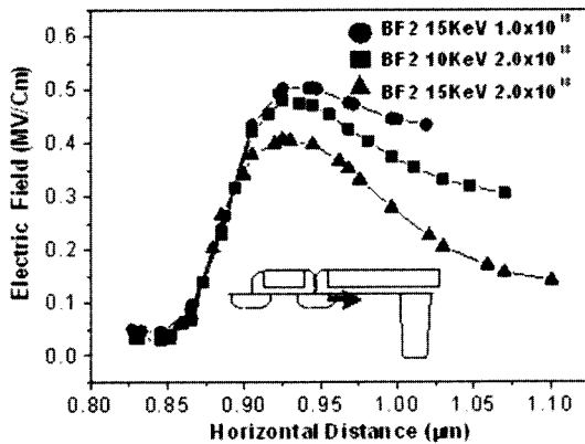
그림 3. 커패시터 V_T 이온주입 조건에 따른 커패시터 아래 계면을 따라 모의 실험한 전장의 세기 분포. Fig. 3. Simulated electric field distribution along horizontal length under the capacitor with different condition of capacitor V_T implant.
