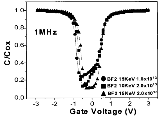
그림 4. 평면구조 P-MOS 커패시터에 대해 1 MHz에서 모의실험한 고주파 C-V특성 곡선. Fig. 4. High frequency C-V characteristics curves, which is simulated at 1 MHz, for planar P-MOS capacitor.
