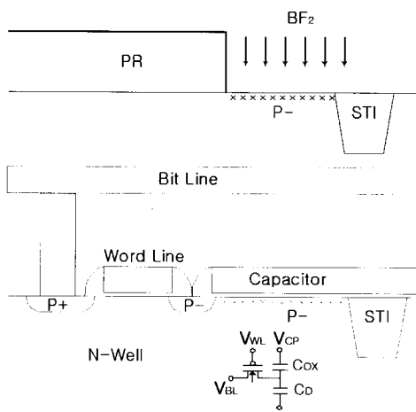
그림 1. 평면구조 P-MOS DRAM 셀의 주요 제조 공정 및 단면구조.
