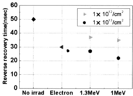
그림 8. 양성자 주입 에너지와 도즈에 따른 역방향 회복 시간.
