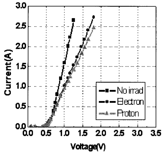
그림 4. 높은 전력에서 순방향 전류-전압 특성.
