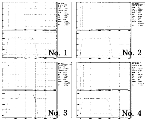
그림 3. 장시간 방전내량시험 파형.
