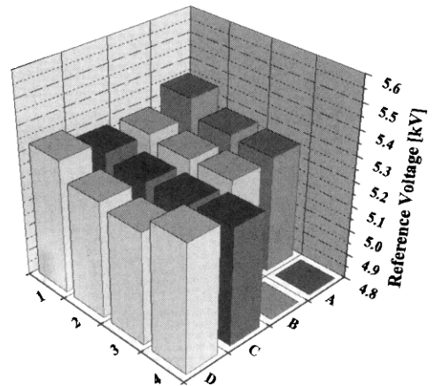
그림 5. ZnO 소자 각 부위의 동작개시전압.
