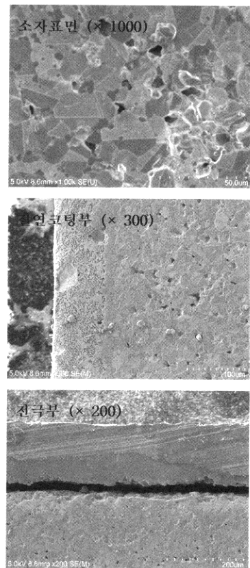
그림 6. ZnO 소자 표면의 미세구조 사진.
