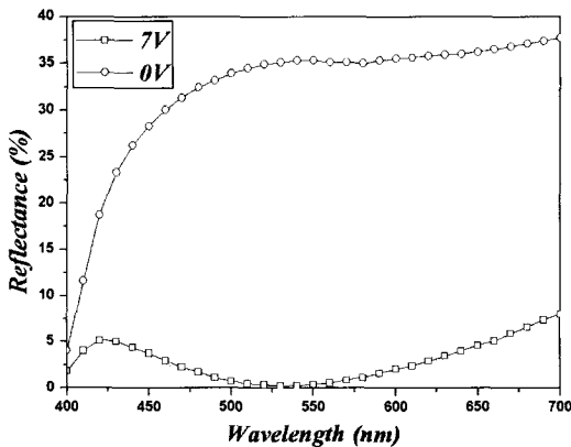
그림 4. 밝음 상태와 어둠 상태의 입사파장에 따른 반사율.
