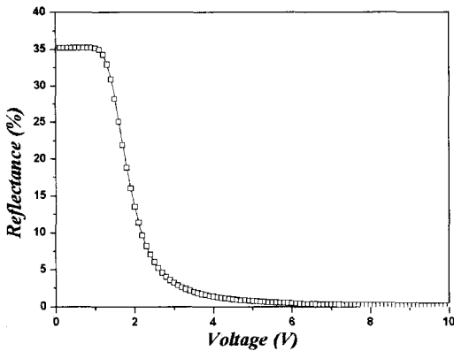
그림 3. 입사파장이 550 nm일 때에 전압인가에 따른 반사율.
