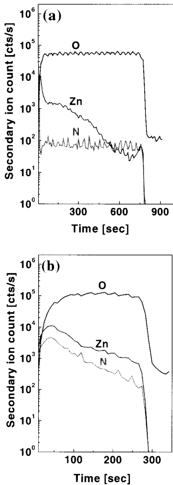
그림 4. ZnO 박막의 Zn, O, N 원소에 대한 atomic profile : (a) as dep. ZnO, (b) NH 3 분위기에서 700 °C 온도로 1 시간 동안 열처리되고 N 2 분위기에서 800 °C 온도로 30 분 동안 열처리(활성화 열처리)된 ZnO 박막.
