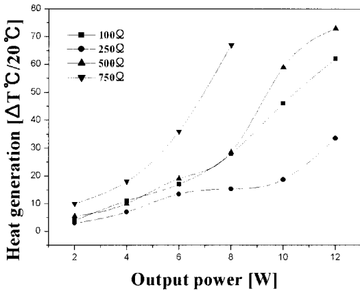
그림 11. 출력전력에 따른 발열.
