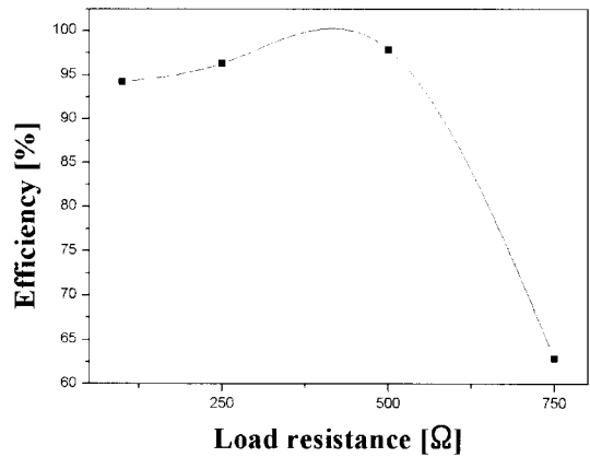
그림 9. 부하저항에 따른 효율. Fig. 9. Efficiency according to load resistance.
