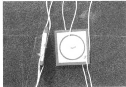
(b) 제작된적층압전변압기
