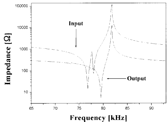
그림 7. 적층 압전변압기의 임피던스특성. Fig. 7. Impedance characteristic curve of multi-layer PT.
