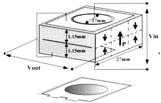
Internal electrode pattern (a) 적층압전변압기구조 및 내부전극 패턴
