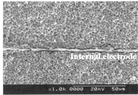
그림 6. 적층 압전변압기의 내부전극과 세라믹스 계면. Fig. 6. Internal electrode and ceramic interfacial surface of multilayer PT.
