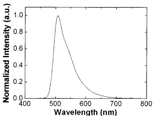
그림 7. 상온에서 PC 기판 상에 제작된 IZO 애노드를 가진 유기물 플렉서블 디스플레이의 EL 스펙트럼.
