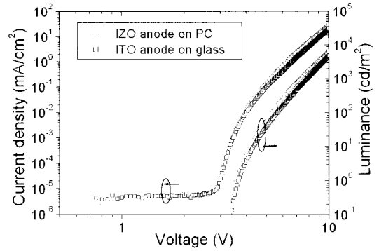
그림 6. IZO/PC와 ITO/glass 기판 상에 제작된 유기물 플렉서블 디스플레이의 전압-전류-휘도 특성.
