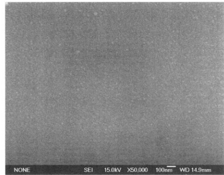
그림 4. 상온에서 PC 기판 위에 성막한 비정질 IZO 애노드 박막의 SEM 표면 이미지.
