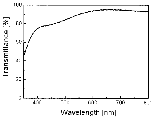
그림 3. 상온에서 PC 기판 위에 성막한 비정질 IZO 애노드 박막의 투과도.
