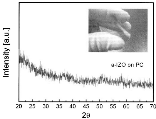
그림 1. DC 스퍼터를 이용하여 상온에서 PC 기판 상에 성막한 IZO 박막의 XRD결과와 사진.
