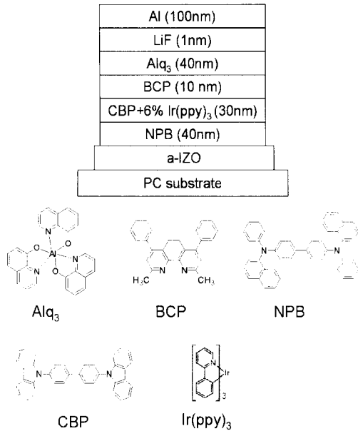
그림 5. PC 기판위에 성막한 비정질 IZO 애노드 상에 제작된 유기물 플렉서블 디스플레이의 구조와 유기물 구조.
