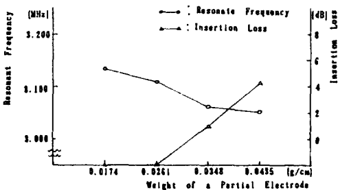
그림 3. 부분전극의 무게에 따른 에너지포획형 공진자의 삽입손실과 공진주파수의 변화 Fig 3. Changes of the insertion loss and the resonant frequency its partial electrode
