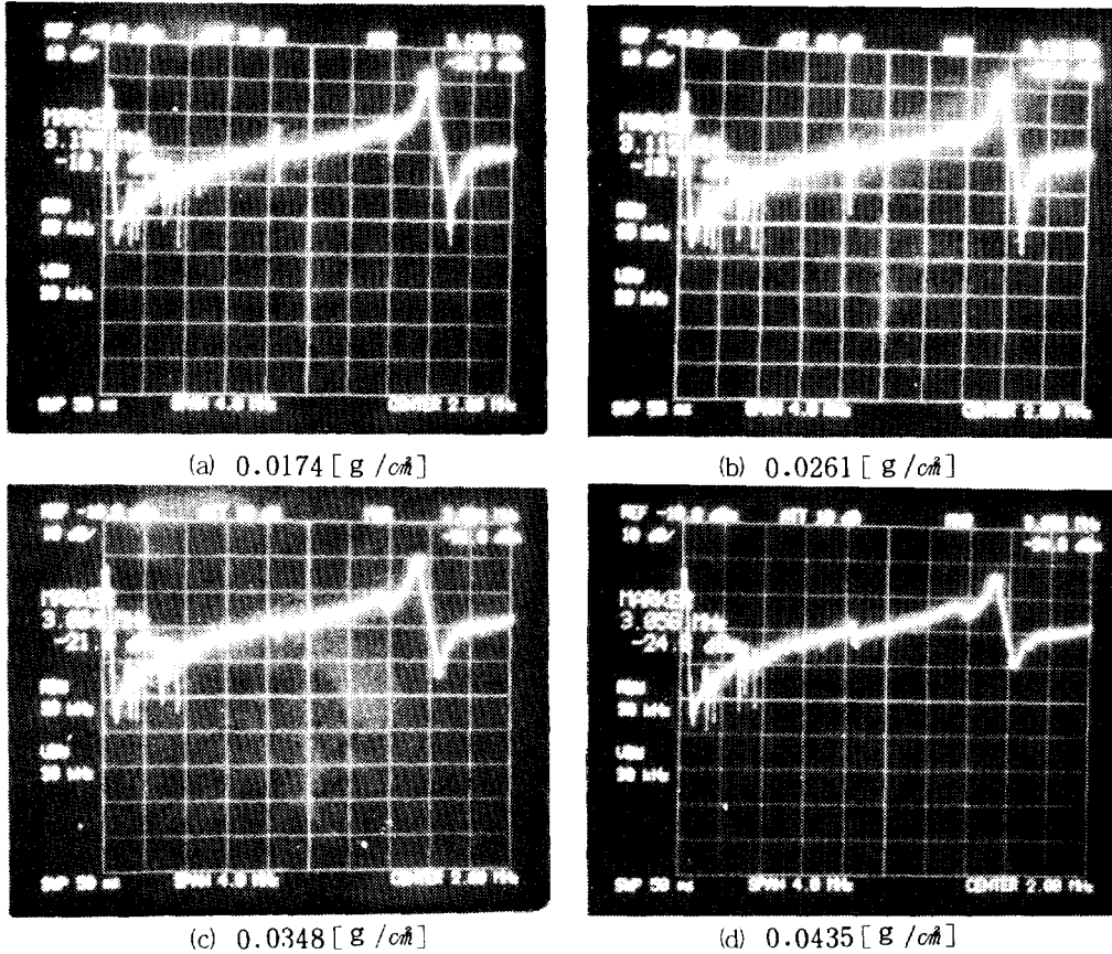
그림 2. 부분전극의 무게에 따른 에너지포획형 공진자의 주파수특성 변화 Fig 2. Frequency characteristic changes of the energy-trapped resonator increasing its partial electrode weight
