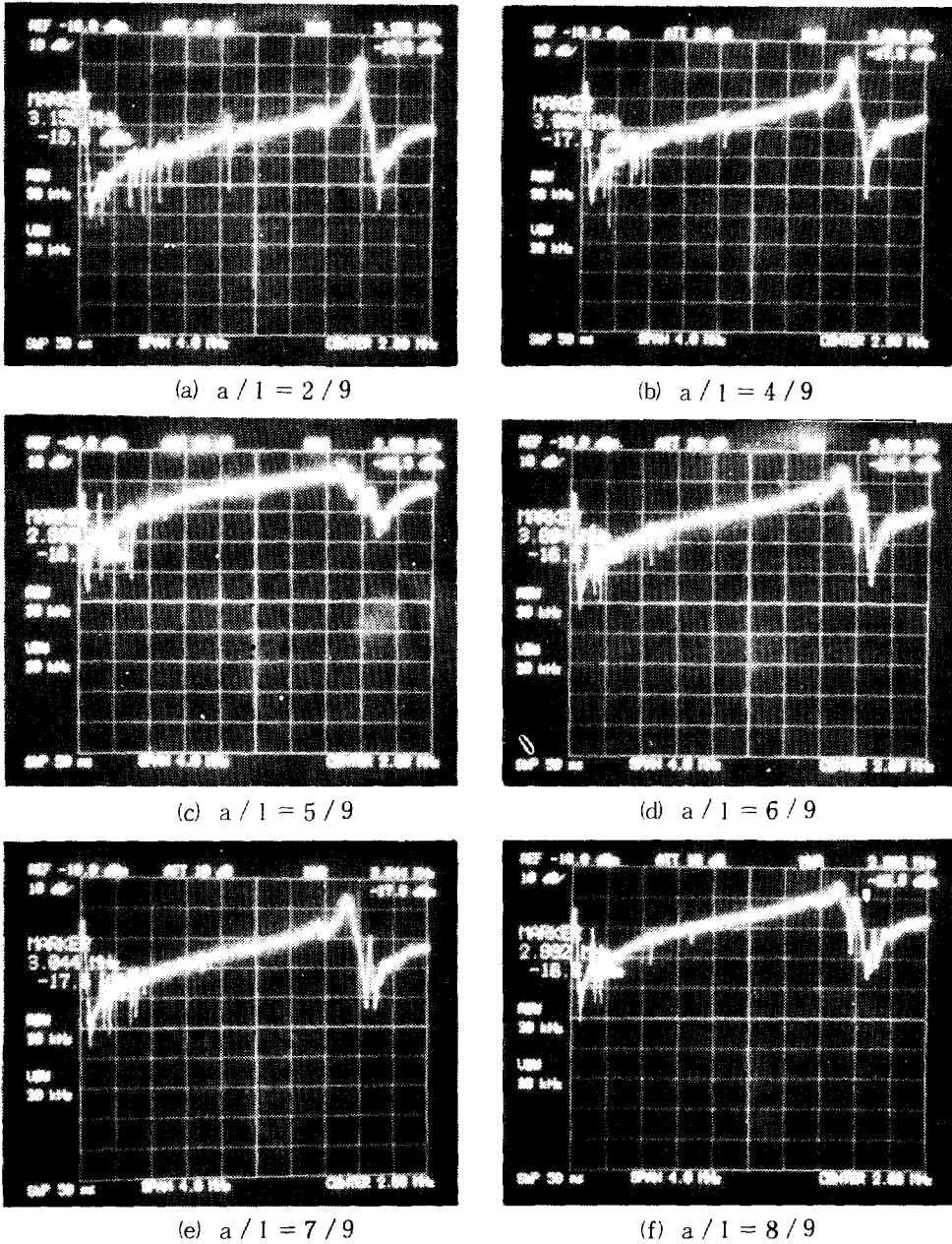
그림 4. 부분전극의 면적 확장에 따른 에너지 포획형 공진자의 주파수특성 변화 Fig 4. Frequency characteristic changes of the energy-thapped resonator according to expanding the area of its partial electrode
