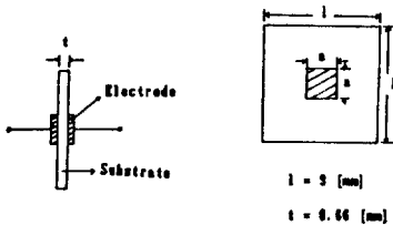
그림 1. 에너지포획형 공진자의 구조
