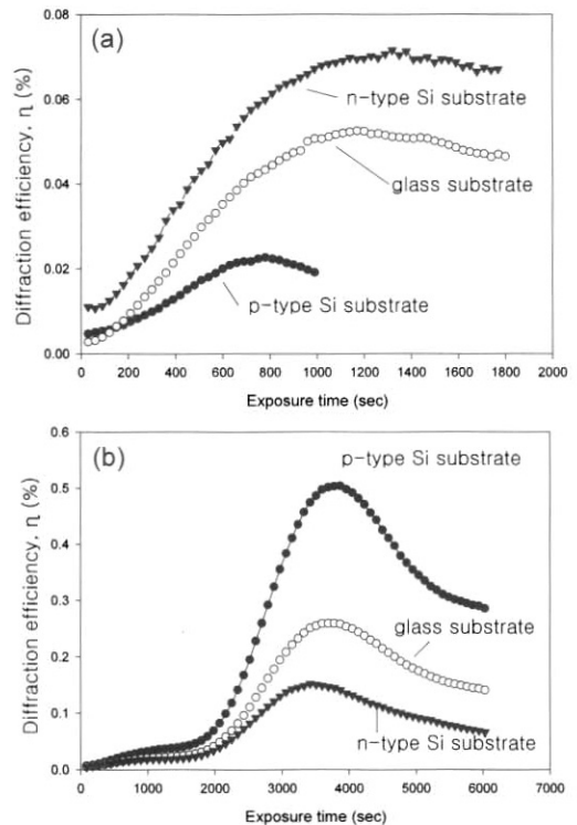
그림 3. 기관의 종류를 달리하여 제작된 (a) type I 및 (b) type II 시료에 대한 회절효율 변화.
