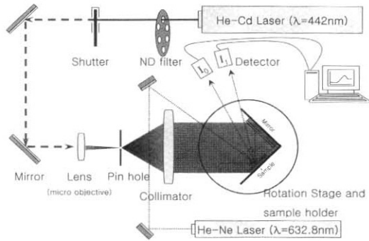
그림 2. 홀로그래피를 위한 노광장치와 실시간 회절효율 측정장치의 개략도.
