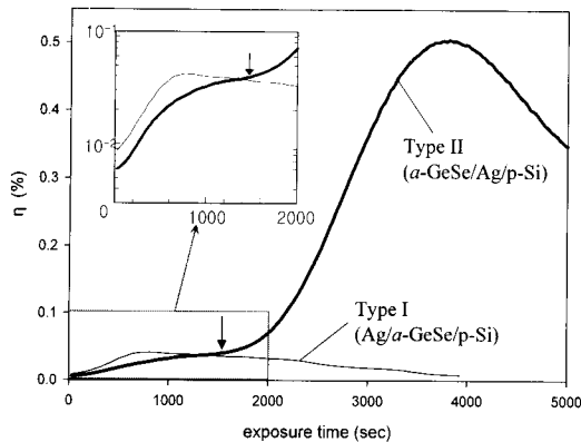
그림 4. p-type Si 기판을 사용한 type I과 type II 시료의 회절효율 변화. 내부 그림은 t = 0 \sim 2000 s에 대한 준 로그 스케일로 표시한 그림이다.
