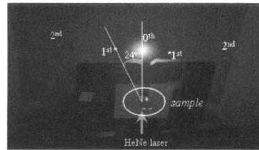
(a) 투과형 회절패턴
