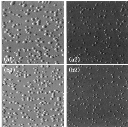
그림 1. InAs 양자점들의 열처리 전후의 AFM 이미지(1 \mu\text{m} x 1 \mu\text{m} ).
