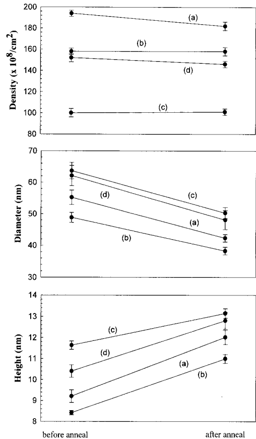
그림 2. 열처리 전후 InAs 양자점들의 밀도 및 크기 변화.
