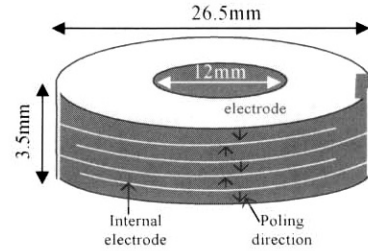
(a) 원환형 적층 압전 액츄에이터의 개략도 5층
