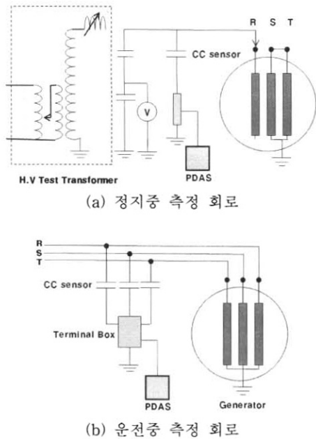
그림 1. 고전압회전기의 운전중 및 정지중 PD 측정회로. Fig. 1. Test circuits of on-line & off-line PD in high voltage rotating machine.
