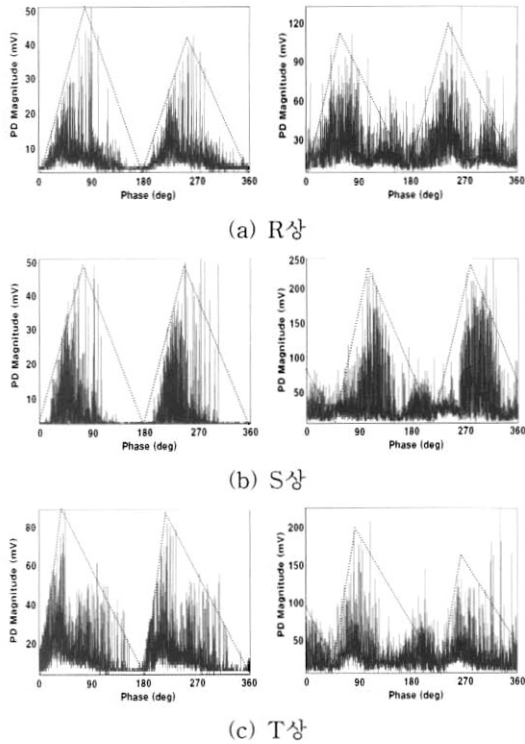
그림 4. 발전기 고정자권선의 상별 PRPD(좌:정지중 시험, 우:운전중 시험).
