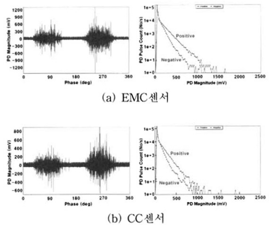
그림 3. 모의슬롯 결합권선의 EMC센서와 CC센서 PD특성. Fig. 3. PD characteristics of EMC & CC sensor for simulated slot defect winding.
