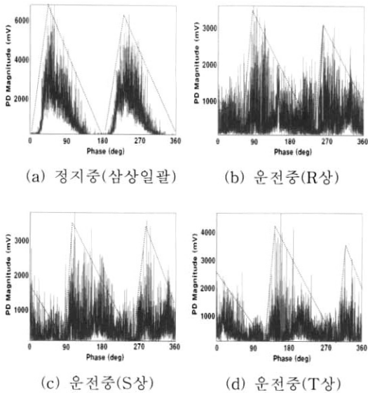
그림 7. 전동기 고정자권선의 PRPD(정지중:삼상일괄, 운전중:상별측정). Fig. 7. PRPD of motor stator windings (off-line: three-phase, on-line: per phase).
