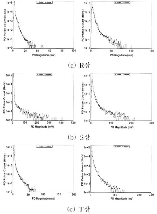
그림 5. 발전기 고정자권선의 상별 PD크기에 대한 PD개수(좌:정지중 시험, 우:운전중 시험).
