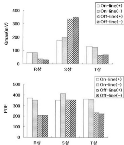
그림 6. 발전기 고정자권선의 Qmax 와 POE.
