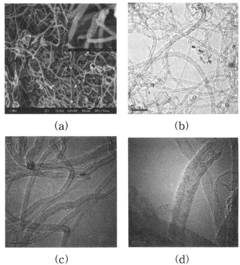
그림 2. 플라즈마 처리 전 탄소나노튜브의 미세 구조: (a) SEM 사진, (b)~(d) TEM 사진.
