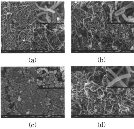
그림 3. 산소 플라즈마 처리에 따른 탄소나노튜브의 미세 구조: (a) 100 Watt, (b) 200 Watt, (c) 300 Watt (표면), (d) 300 Watt (내부).
