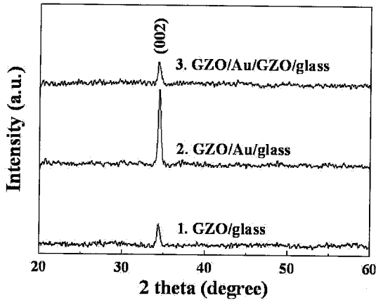
그림 1. Au 금속층을 이용한 투명전도막의 XRD 패턴.
