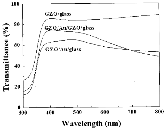
그림 3. Au 금속층을 이용한 투명전도막의 광투과도.
