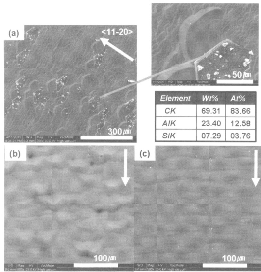
그림 3. SiC/Al 분말 비율에 따라 성장된 p-type 에피텍셜층의 결함 및 표면 형상을 전자현미경으로 관찰. (a) SiC/Al=20/1 비율로 성장된 에피텍셜층의 결함 관찰 및 성분 분석 (b) SiC/Al=30/1 (c) SiC/Al=50/1
