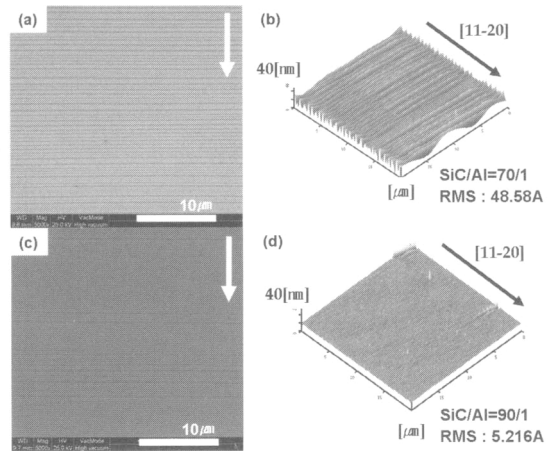
그림 4. SiC/Al 분말 비율에 따라 성장된 p-type 에피텍셜층의 표면 형상을 전자현미경 관찰 및 AFM 결과. (a) SiC/Al=70/1 (b) SiC/Al=70/1 AFM 결과 (c) SiC/Al=90/1 (d) SiC/Al=90/1 AFM 결과
