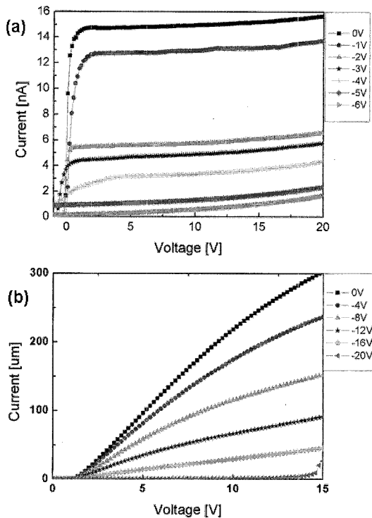
그림 6. 게이트 거리가 20 \mu\text{m} 와 40 \mu\text{m} 일 때 MESFET의 I-V 특성. (a) 게이트 전압이 0 V이고, 드레인 전압이 5 V일 때 전류는 15 nA에서 포화되었다. (b) 게이트 전압이 -20 V일 때 더 이상 전류는 흐르지 않았다.
