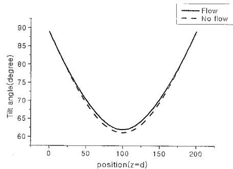
그림 6. VA-LCDs에서 switching off 이후 30 msec에서의 분자배열 분포.
