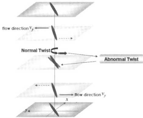
그림 4. Switching off 상태에서 흐름효과를 고려한 IPS-LCDs의 액정 분자 거동 모식도.
