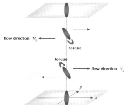
그림 7. Switching off 이후 흐름효과를 고려한 VA-LCDs의 액정 분자 거동 모식도.
