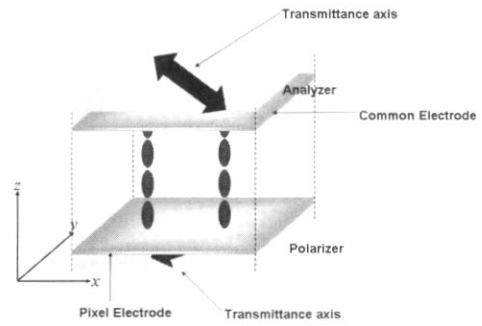
그림 5. VA-LCDs 시뮬레이션을 위한 좌표계의 정의 및 초기조건.
