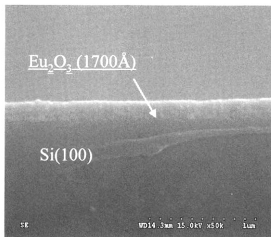
그림 1. p-type Si(100) 기판 상에 증착된 유로퓸-산화막 박막의 주사 전자 현미경 단면사진.
