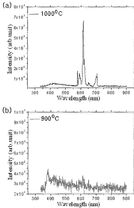
그림 4. 산소 분위기에 따른 1000 °C(a)와 900 °C (b)에서 5분 동안 열처리한 시편에 325 nm He-Cd 레이저를 사용하여 측정된 PL 스펙트럼 분석 결과.
