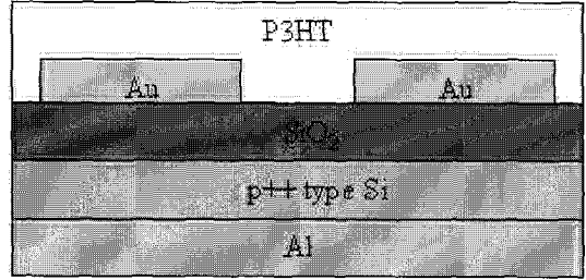
그림 1. 하부 전극 구조의 OTFT. Fig. 1. OTFT with Bottom Contact (BC) configuration.
