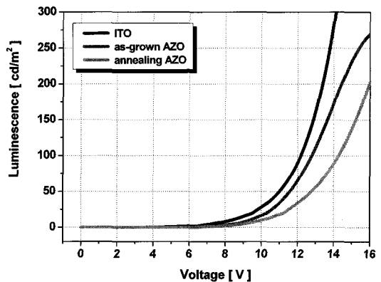
그림 6. AZO와 ITO anode를 적용한 OLED 소자의 휘도-전압 특성. Fig. 6. The luminescence-voltage characteristics of OLED with AZO and ITO anode electrodes.
