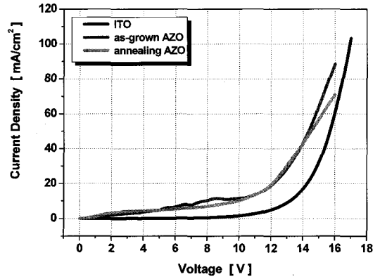
그림 5. AZO와 ITO anode 전극이 적용된 OLED의 전류-전압 특성. Fig. 5. The current density-voltage characteristics of OLED with AZO and ITO anode electrodes.
