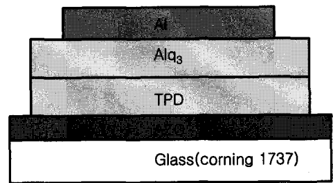
그림 1. OLED 소자의 구조 모식도. Fig. 1. Structural drawing of OLED devices.
