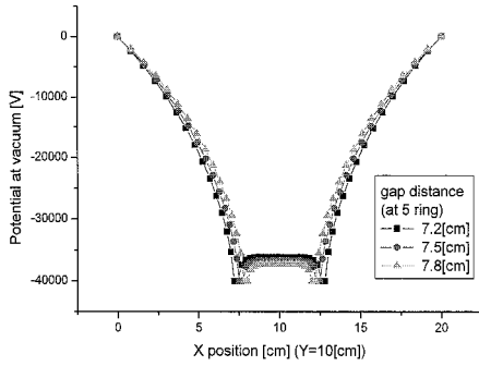
그림 8. 갭 길이의 변화에 따른 진공에서 포텐셜 분포. Fig. 8. Potential distribution with changing gap distance at vacuum.
