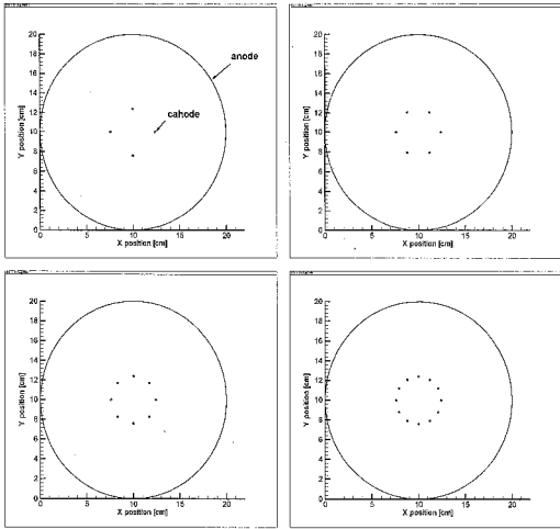
그림 2. 링의 개수에 따른 SCBF 장치의 해석모델 (왼쪽 위부터 3링, 4링, 5링, 6링 구조). Fig. 2. Analysis model according to the number of rings.
