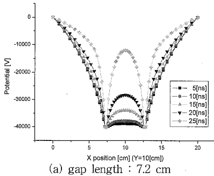
그림 8. 갭 길이의 변화에 따른 진공에서 포텐셜 분포. Fig. 8. Potential distribution with changing gap distance at vacuum.
