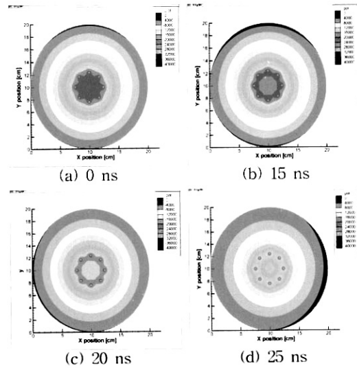
그림 6. 5링 구조에서 포텐셜 분포. Fig. 6. Potential distribution at 5 ring geometry.
