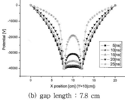
그림 9. 갭 길이를 변화시킬 때 5링 구조의 중심 축에서 포텐셜 분포. Fig. 9. Potential distribution at 5 ring geometry on axis.
