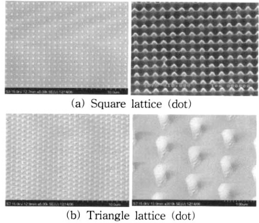
그림 6. dot 형태의 (a) 사각 및 (b) 삼각 격자구조의 2차원 광자결정 배열에 대한 SEM 이미지.
