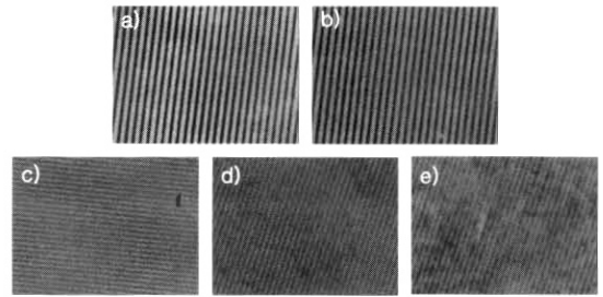
그림 3. 폴리머 레지스트의 홀로그래피에 의해 형성된 직선 격자의 광학현미경 이미지. 노광시간 = t_{max} ; 현상시간 = 15초; 레이저 파워밀도(mW/cm 2 ) = (a)30, (b)50, (c)60, (d)80, (e)100.
