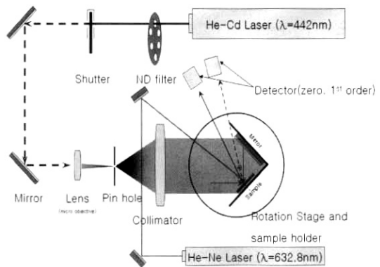
그림 1. 홀로그래피를 위한 노광장치와 실시간 회절효율 측정장치의 개략도.
