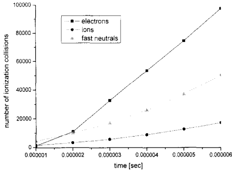
그림 9. 5링 구조에서 각 입자들의 전리충돌 수. Fig. 9. The number of ionization collisions at 5 ring geometry.
