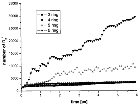
그림 4. D_2^+ 이온의 수.
