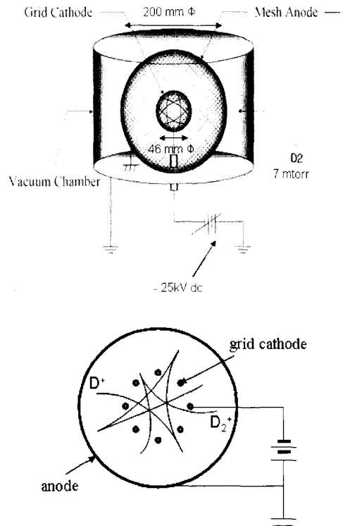
그림 1. SCBF 장치의 구성도 및 이온의 운동. Fig. 1. Schematic of SCBF device and the motion of ions.
