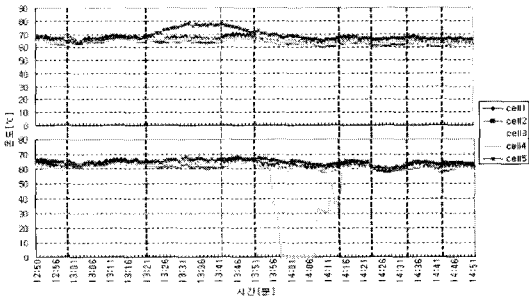
그림 6. 옥외 설치 시 그림자 영향에 의한 태양전지 모듈의 시간 흐름에 따른 온도 변화. Fig. 6. Temperature variation with time by shading effect for outdoor system.
