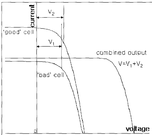
그림 1. 직렬 연결된 미스매치 태양전지가 전압에 미치는 영향.
