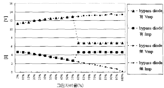
그림 8. 그림자 비율(%)과 bypass diode 유·무에 따른 태양전지 모듈의 Vmp, Imp 값의 변화. Fig. 8. Vmp and Imp variation with shading ratio(%) with and without bypass diode.
