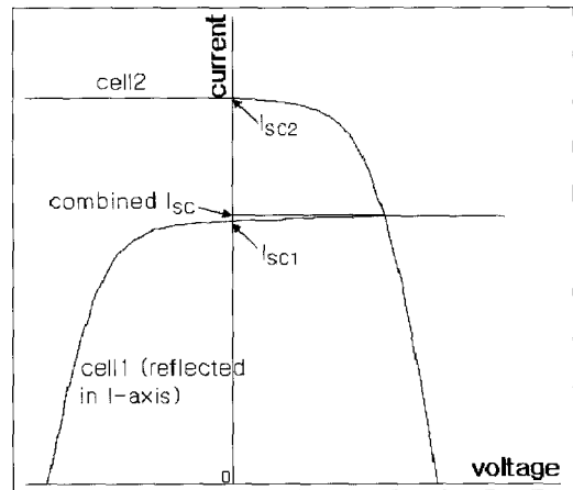
그림 2. 직렬 연결된 미스매치 태양전지의 합성 전류( I_{sc} ).
