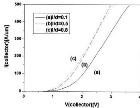
그림 4. 트랜치 IGBT의 I-V 특성곡선. Fig. 4. I-V characteristics for Trench IGBT.
