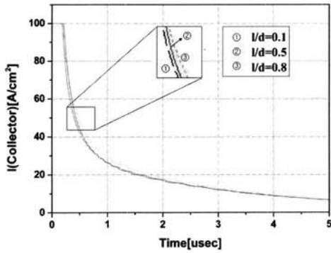
그림 5. 트랜치 IGBT의 턴-오프 시뮬레이션 결과. Fig. 5. Turn-off simulations of Trench IGBT.
