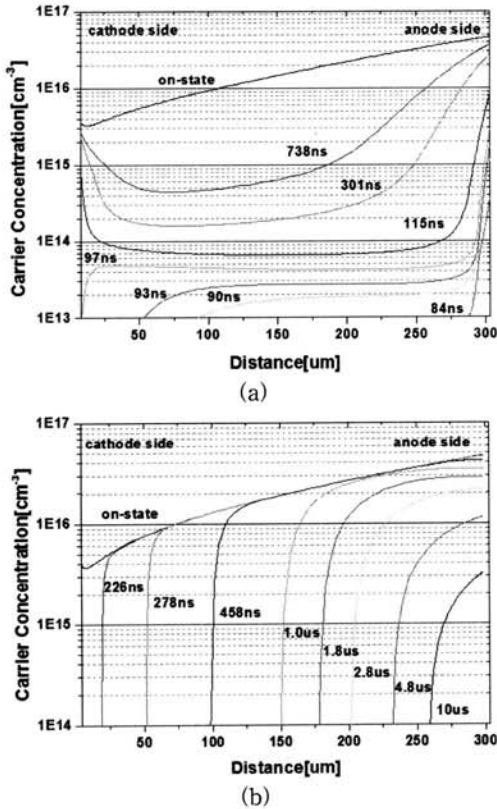
그림 6. 스위칭시 트랜치 IGBT의 n-드리프트 영역에 대한 전자 분포. (a) 턴-온 스위칭시 (b) 턴-오프 스위칭시. Fig. 6. Electron distribution in the n-drift of a Trench IGBT during switching. (a) during turn-on switching (b) during turn-off switching.
