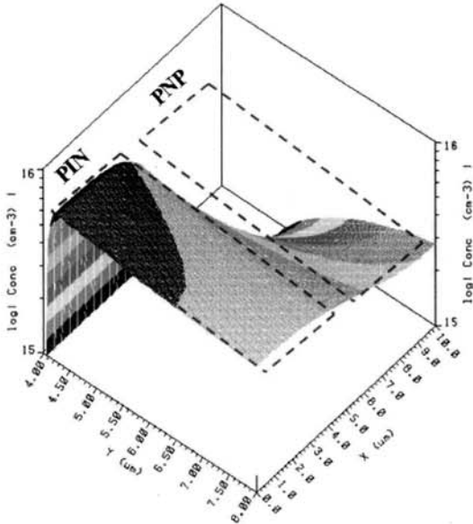
그림 2. 트랜치 IGBT 캐소드측에서의 캐리어 분포. Fig. 2. Carrier distribution at the cathode side in the Trench IGBT.
