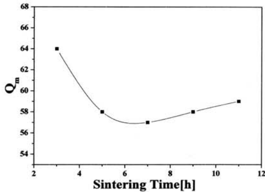
그림 5. 소성시간 변화에 따른 기계적품질계수(Q m ). Fig. 5. Mechanical quality factor (Q m ) with variations of sintering time.
