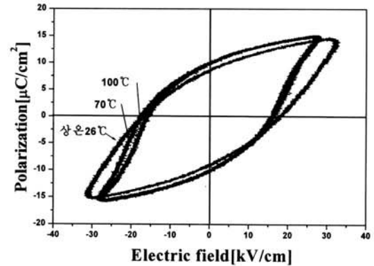
그림 7. 시편의 히스테리시스 곡선. Fig. 7. Hysterisis curve of specimens.
