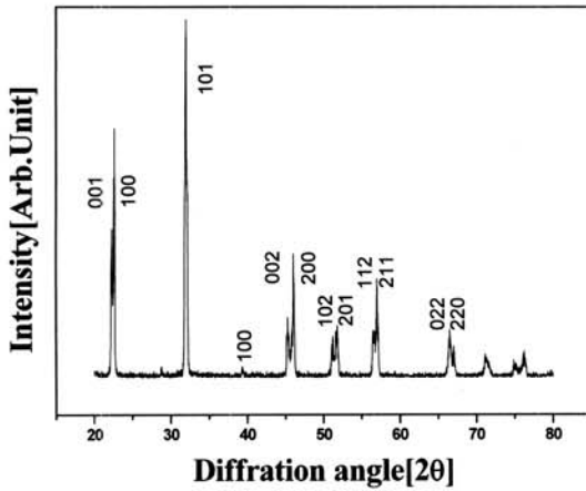
그림 2. X선 회절 패턴. Fig. 2. X-ray diffraction pattern.
