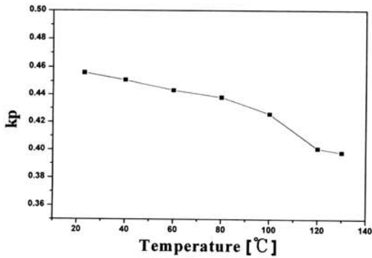
그림 6. 시편의 kp의 온도 의존성. Fig. 6. Temperature dependence of electro-mechanical coupling factor(kp).
