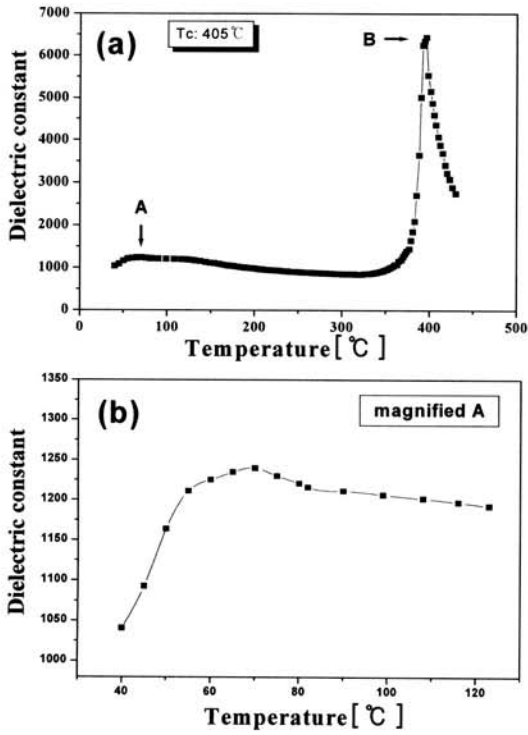
그림 5. 유전상수의 온도의존성(a)과 A부분의 확대(b). Fig. 5. Temperature dependence of dielectric constant(a) and magnified A(b).
