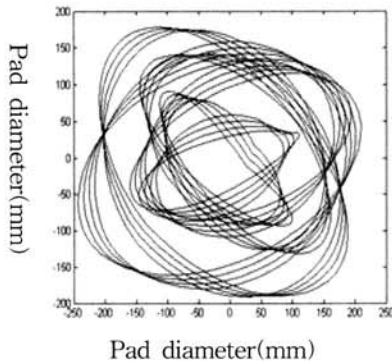
그림 3. 패드상 다이아몬드 입자가 그리는 궤적. Fig. 3. A path drawn by diamond grid on pad.
