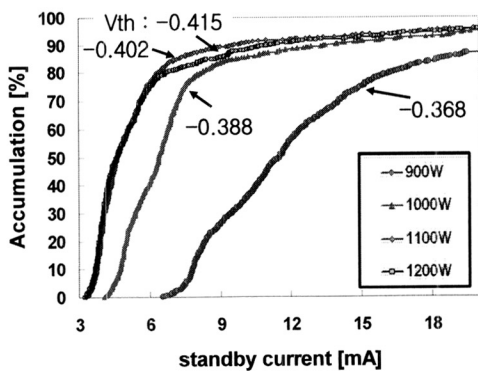
그림 6. DPN power에 따른 standby current. Fig. 6. Standby current with DPN power.
