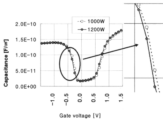
그림 4. DPN power에 따른 PMOS의 C-V curve. Fig. 4. CV characteristics of PMOS with power.
