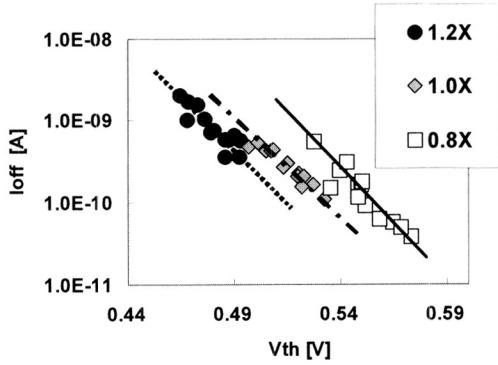
그림 5. DPN power에 따른 NMOS의 I_{off} 특성. Fig. 5. I_{off} of NMOS with DPN RF power.
