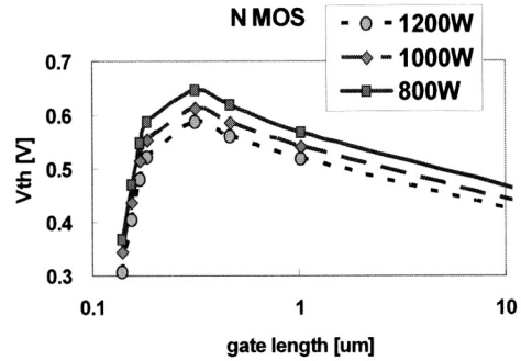
그림 2. DPN power에 따른 NMOS roll off 특성. Fig. 2. NMOS roll off with DPN power.
