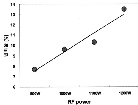
그림 8. DPN RF power에 따른 Fowler-Nordheim stress 후 NMOS TR의 V_{th} 변화율. Fig. 8. V_{th} shift of NMOS TR with DPN RF power after Fowler-Nordheim stress.
