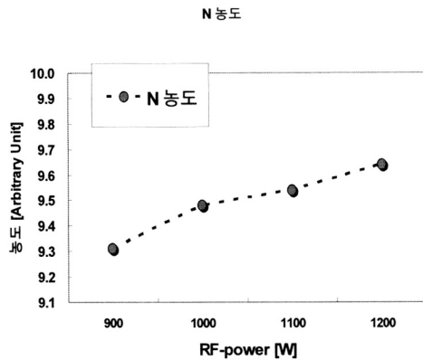
그림 1. 산화물 내 질소 농도. Fig. 1. N concentration in oxide.
