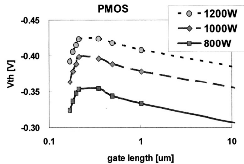
그림 3. DPN power에 따른 PMOS roll off 특성. Fig. 3. PMOS roll off with DPN power.
