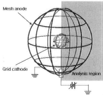
그림 1. 구형 집속 빔 핵융합 장치의 구성도. Fig. 1. Schematic view of spherically convergent beam fusion device.
