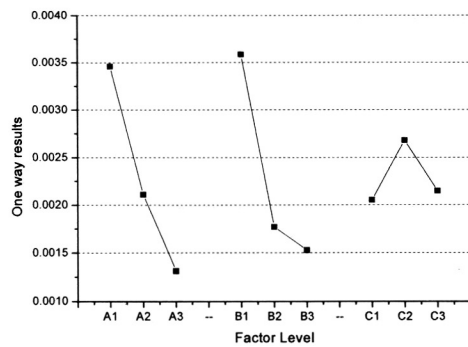
그림 5. 이온전류에 대한 인자수준의 효과. Fig. 5. Effect of factor levels on ion current.
