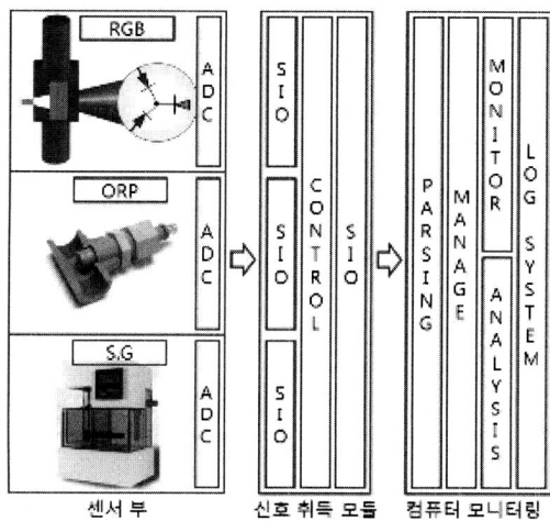
그림 1. 전체 시스템 구성도. Fig. 1. System configuration.
