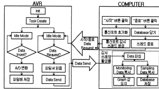
그림 5. 전체 운영프로그램의 구성도. Fig. 5. The configuration of total program.
