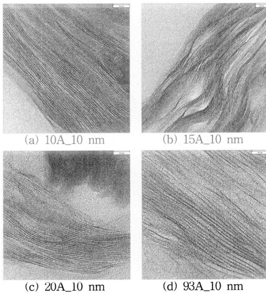
그림 2. 여러종류의 DGEBA/organoclay에 대한 TEM 영상.
