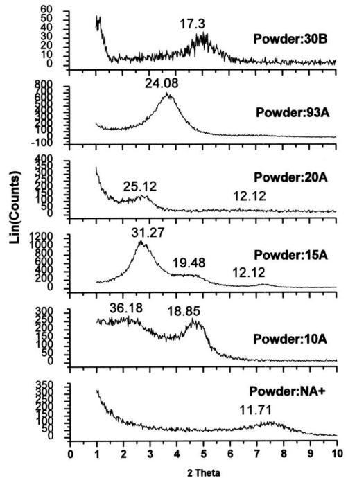
그림 3. 유기화된 크레이 원형파우더의 X-RD.
