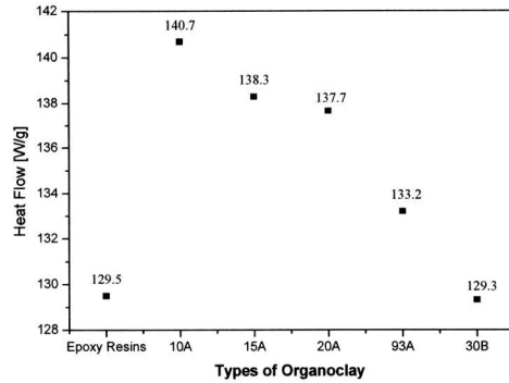
그림 5. Epoxy/organoclay nanocomposites의 DSC 특성.
