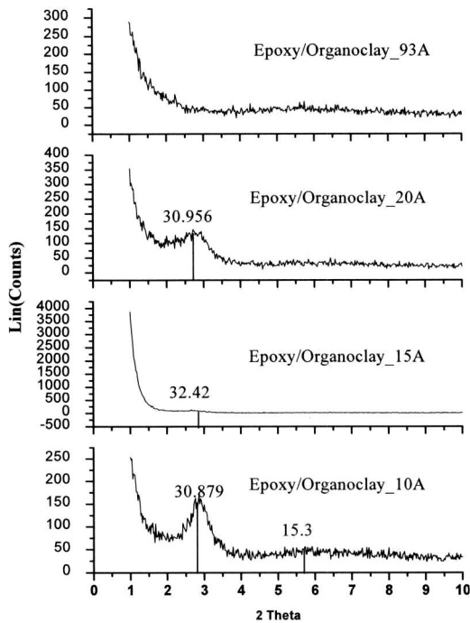
그림 4. 에폭시-유기화된 크레이의 나노복합체의 X-RD 결과.
