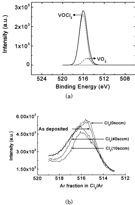
그림 5. (a) V 2p spectra deconvolution (Ar 10 %인 경우). (b) V 2p 스펙트럼 Fig. 5. (a) V 2p spectra deconvolution (Ar fraction = 10 %). (b) V 2p spectrum
