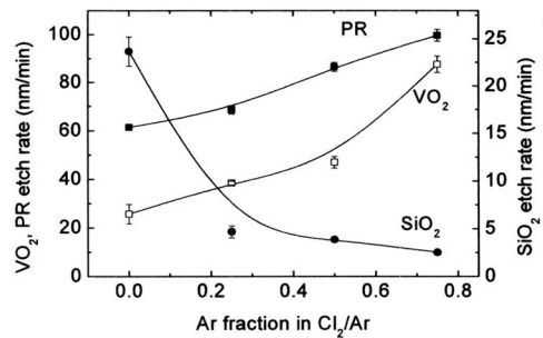
그림 1. 가스 혼합비에 따른 VO 2 박막, SiO 2 , 그리고 감광막의 식각 속도.
